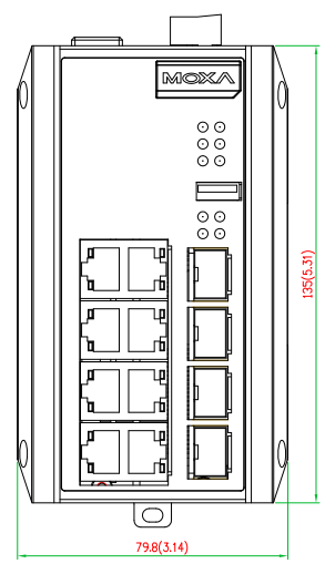
EDS-G512E
