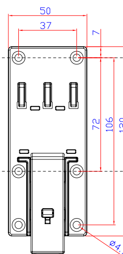
DIN RAIL KIT
