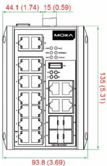
EDS-518E-4GTXSFP
