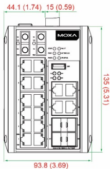
EDS-518E-MM-SC-4GTXSFP/ EDS-518E-SS-SC-4GTXSFP
